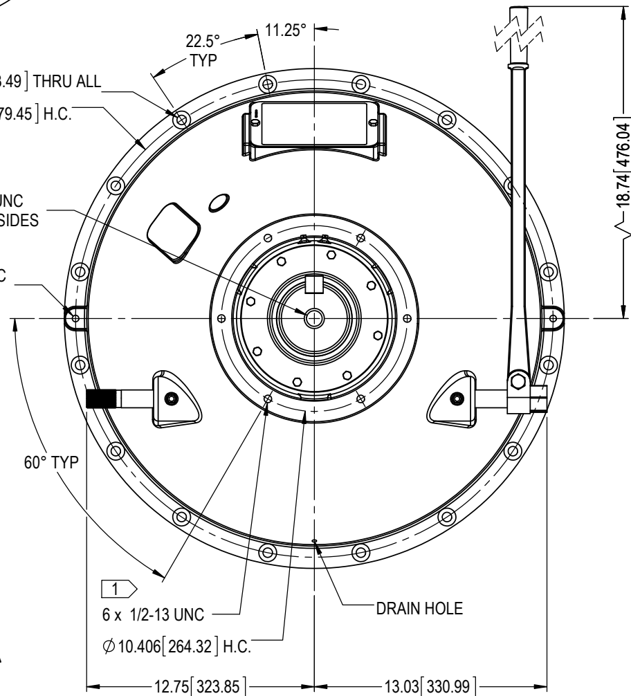
SECTION A-A
